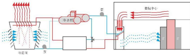
直接蒸发冷却制取冷水整体解决方案原理-板换应用
