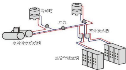
热管背板空调-板换应用
