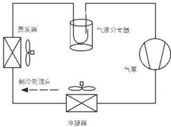
c.气泵动力型
