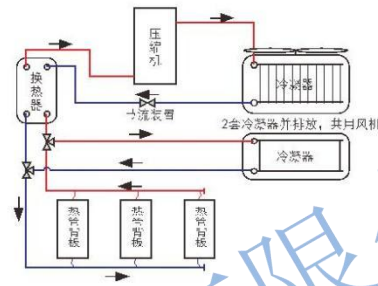
双冷源一体化机房空调+热管背板原理图-板换应用
