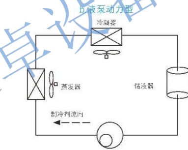
三种分离式热管-板换应用(冷凝器)
